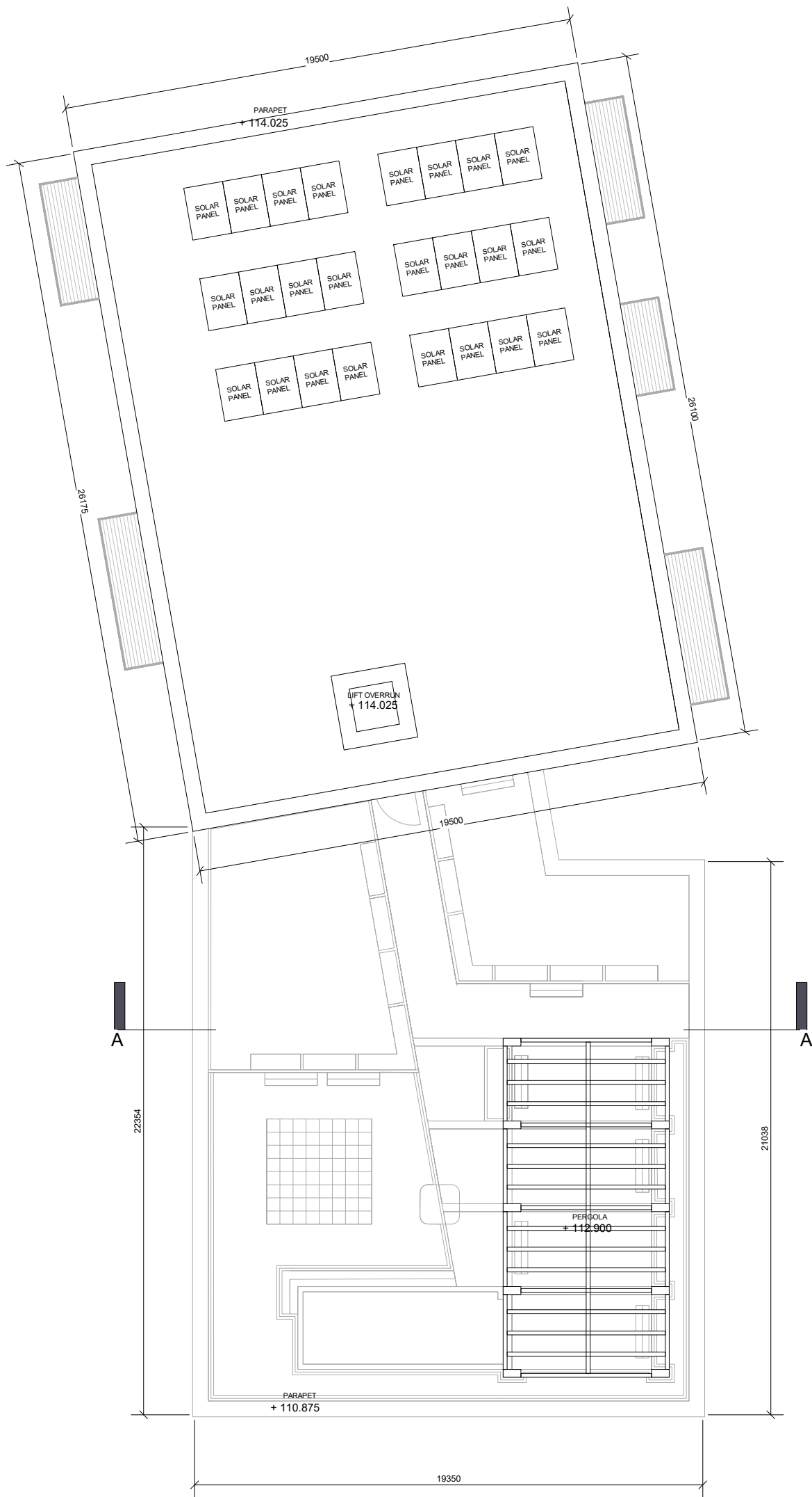
1 Block 01 - Level 05 1 : 200
